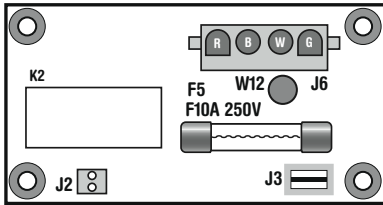
X-B CE N°/P 53311 Utilizado para salida de Compresor SOLAMENTE cuando la Bomba 2 (J5) es una bomba de 2 velocidades. (W15 conectado a J98)
